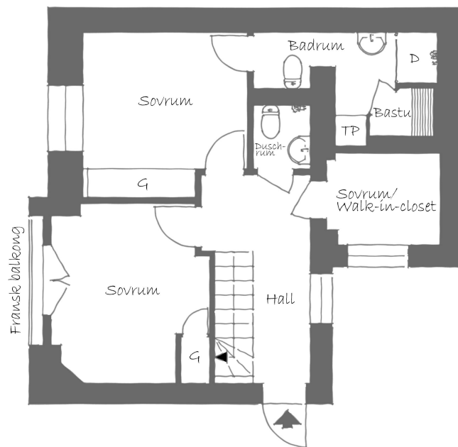
Entréplan
