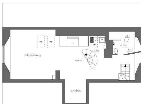
Övre plan
