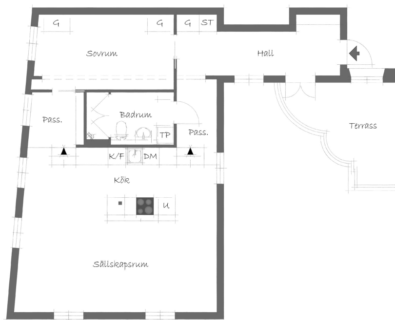
Ateljén Plan 2
